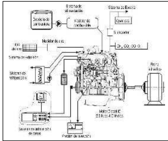
Figura 1. Uso del biodiésel en motores de diésel (Sandoval, 2015) NORMA APA
